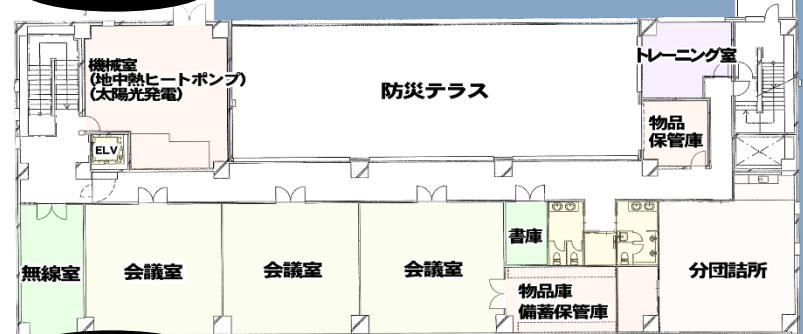
PH 階平面図
